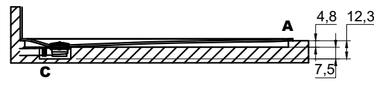
Da appoggio - Top mount
